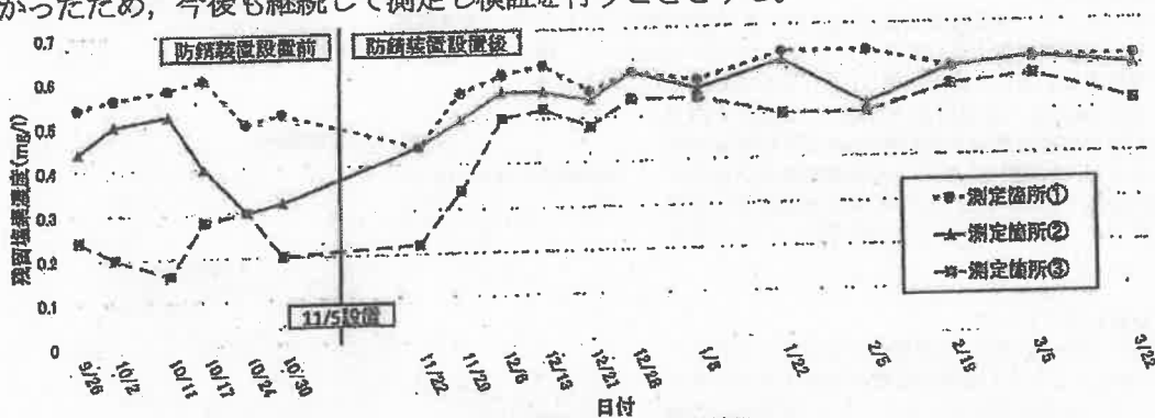
図-3 残留塩素濃度測定結果
