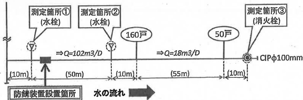
図-2 配管状況及び採水箇所
