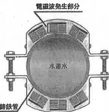
図-1 防錆装置
