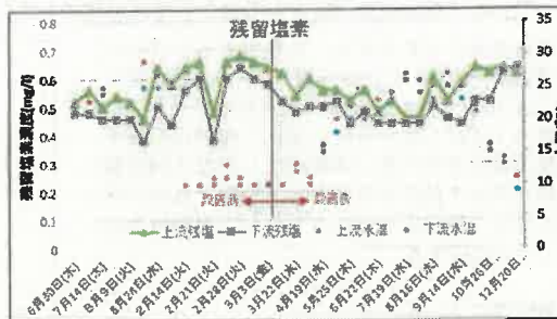
図-5 残留塩素濃度測定結果 (設置場所 NO. 2-港南中央)
