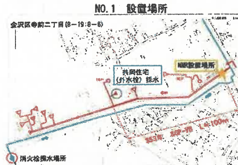
図-2 設置場所 NO.1-寺前二丁目
